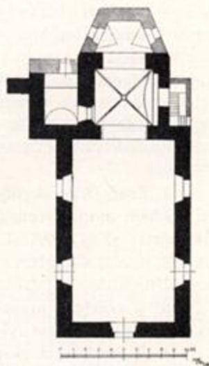
Obr. 5. Běhařov. Půdorys filiálního kostela sv. Prokopa.
